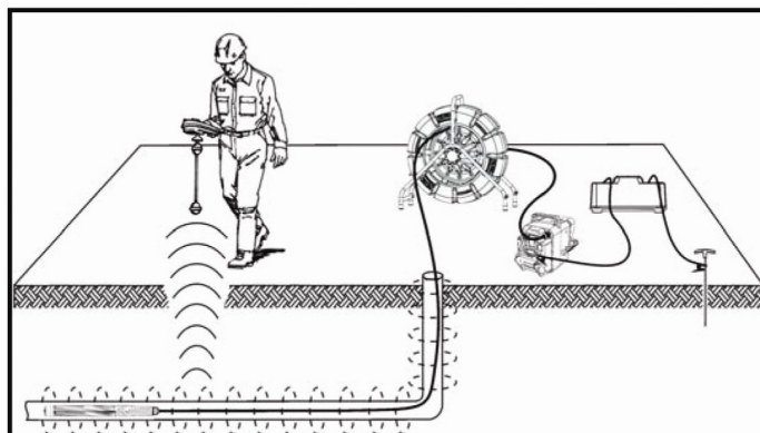
図 11 カメラヘッドケーブルによる経路トレース
