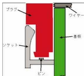
図 27 コネクタの向き
